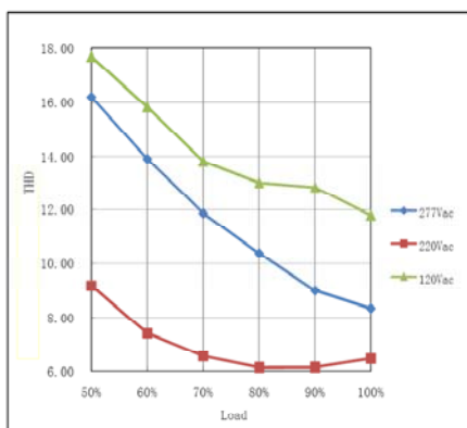
THD Curve(Model:700mA)
