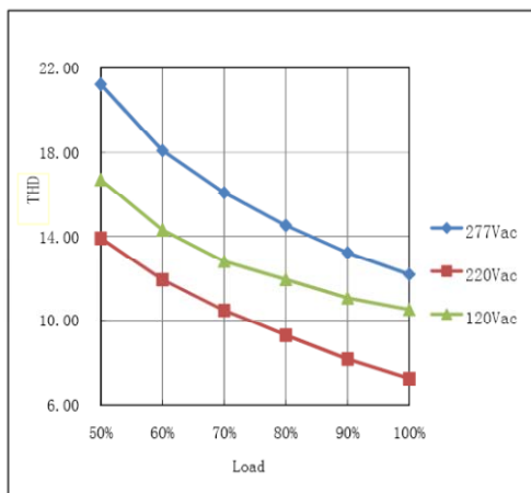
THD Curve(Model:700mA)
