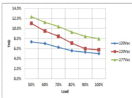
THD Curve(Model:700mA)
