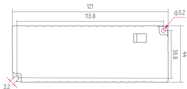
Dimension(mm)
