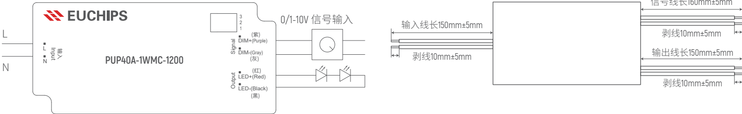
应用接线图
