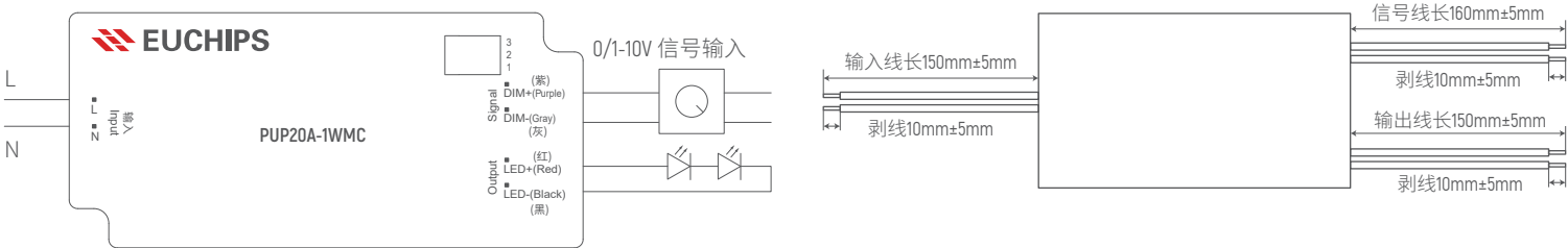
应用接线图
