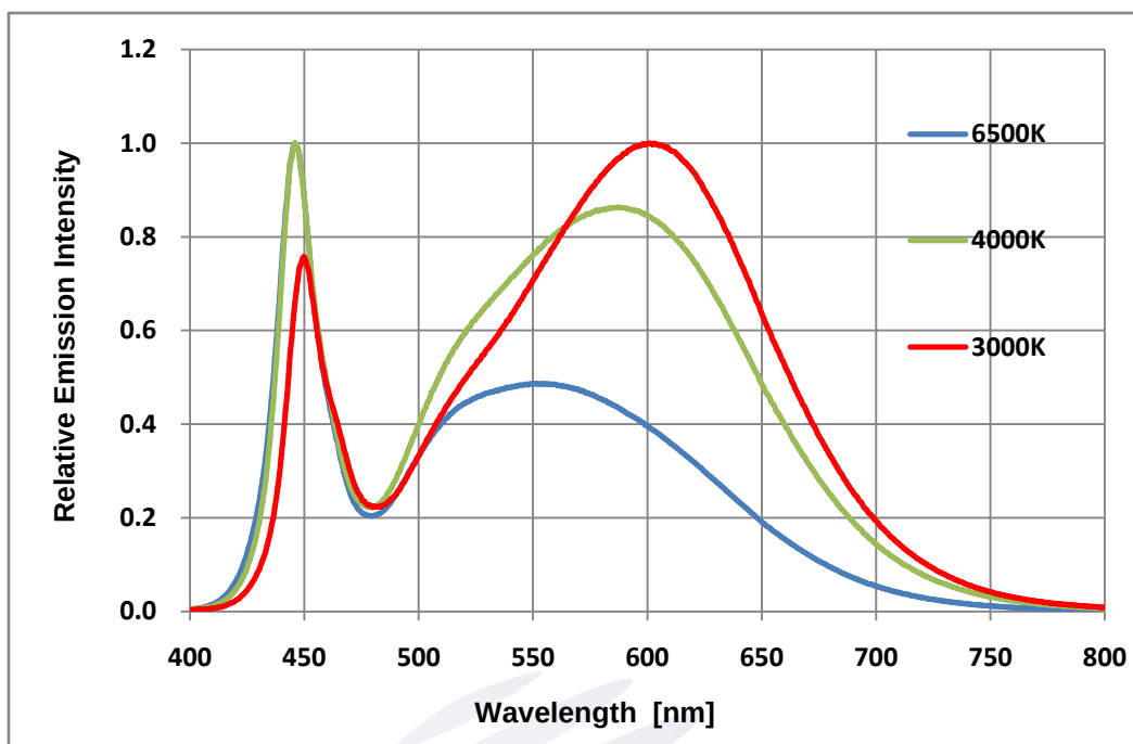
Fig 1-15 Spectrum Distribution光譜分布特性曲线
