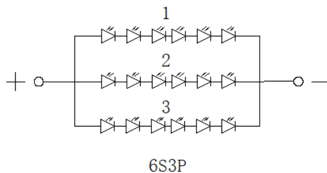
Fig.1-3 Polarity 极性
