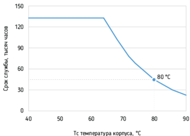
Срок службы
