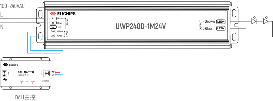
应用接线图
