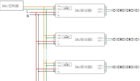
DALI应用图
