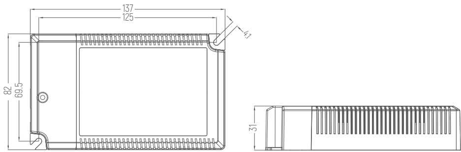
尺寸(mm)
