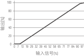
调光曲线
