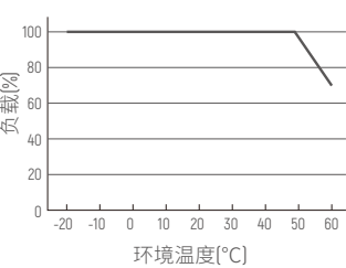
降额曲线
