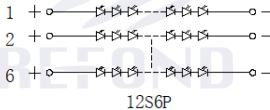
Fig.1-3 Polarity 极性
