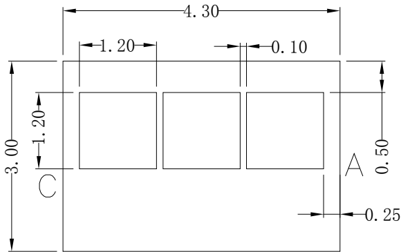
Fig.1-1 Top View 正面视图
