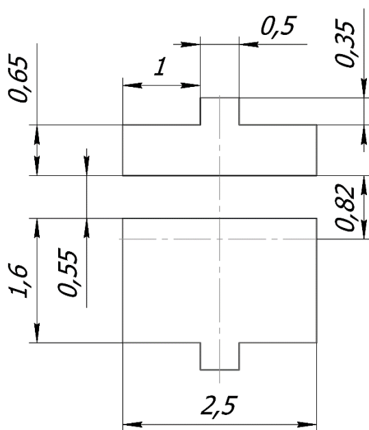
Рекомендуемые размеры контактных площадок
