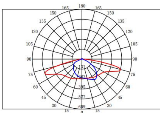
配光曲线
