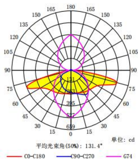
配光曲线
