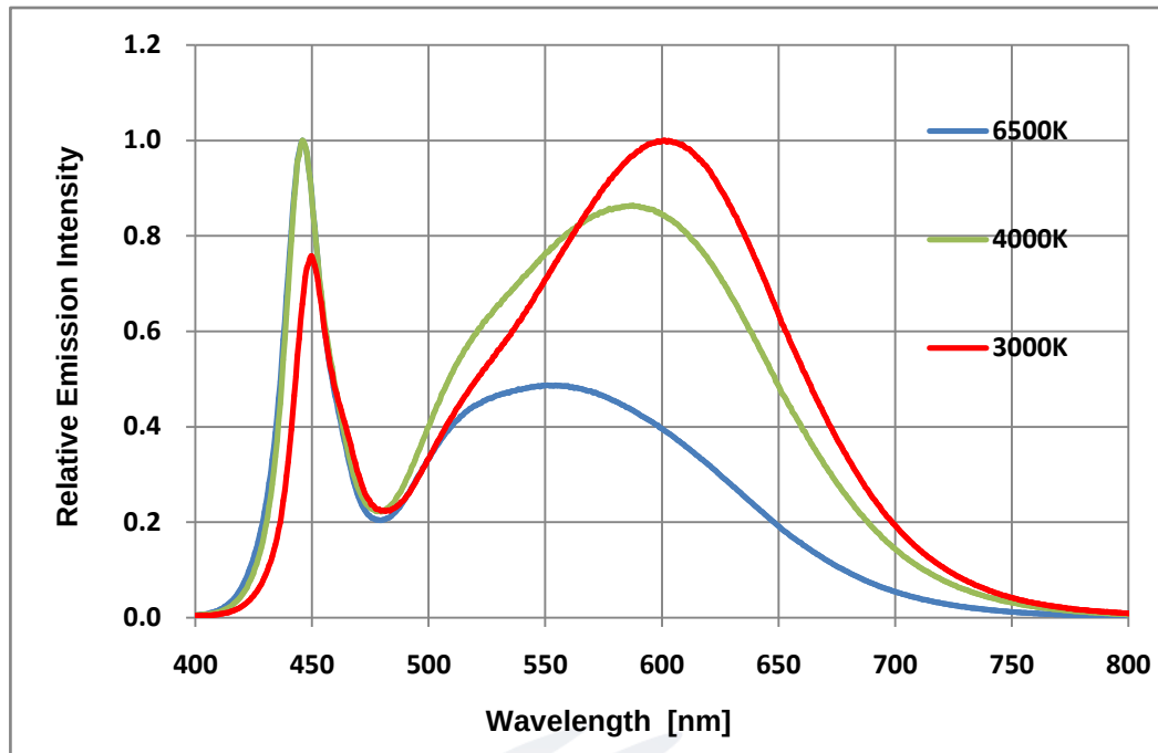
Fig 1-13 Spectrum Distribution光譜分布特性曲线
