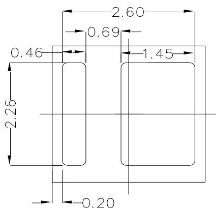
Fig.1-3 Bottom view 背面视图
