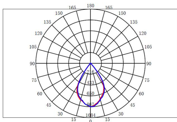
配光曲线
