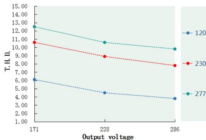
T.H.D. VS Output voltage(DL-200H-286A/P-MXC)
