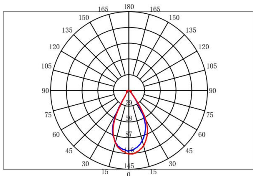
配光曲线
