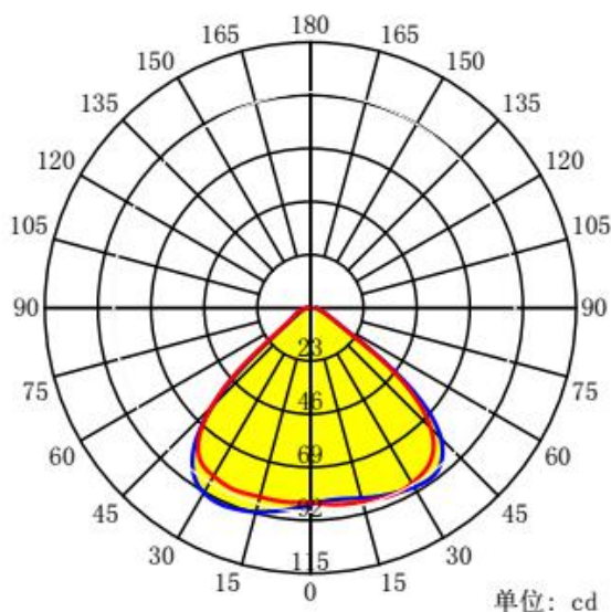
配光曲线
