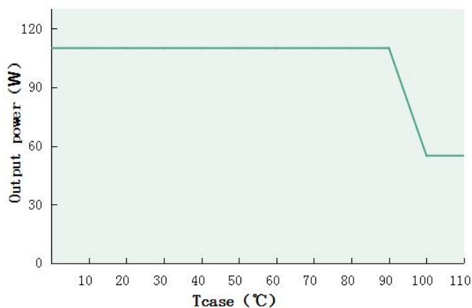
Output power VS Tcase (DL-110H-P/X-MXK)
