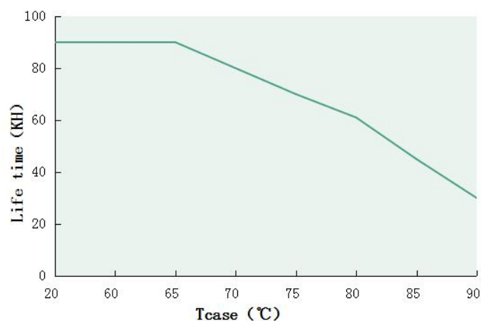
Tcase VS Lifetime (DL-110H-P/X-MXK)
