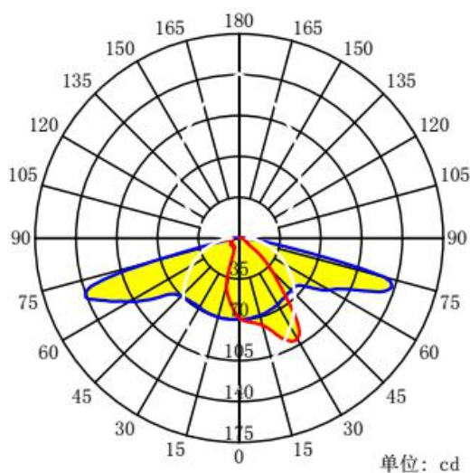
配光曲线
