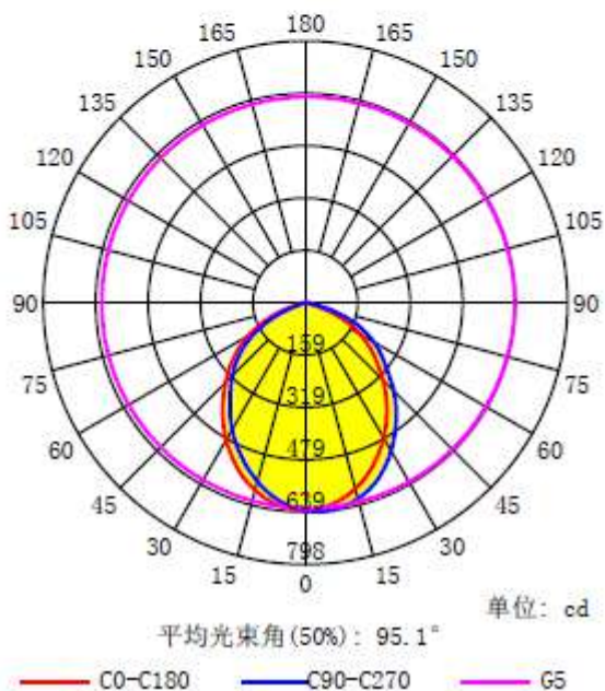
配光曲线
