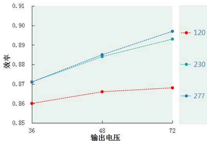
效率 VS 输出电压 DL-50W-V72A/P-MXG
