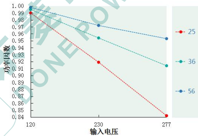
功率因素 VS 输入电压 DL-50W-V56A/P-MXG
