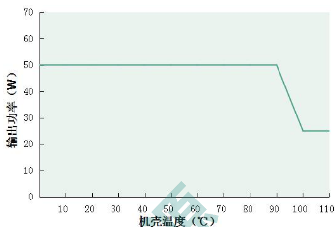
输出功率 VS 机壳温度(DL-50W-A/P-MXG)
