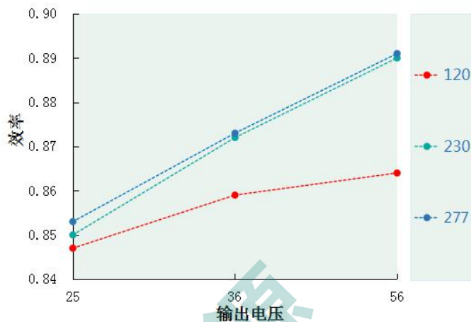
效率 VS 输出电压 DL-50W-V56A/P-MXG
