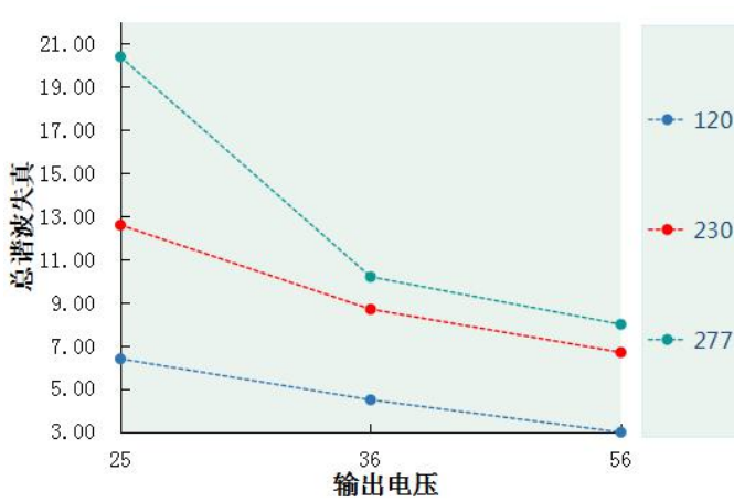
总谐波失真 VS 输出电压 DL-50W-V56A/P-MXG
