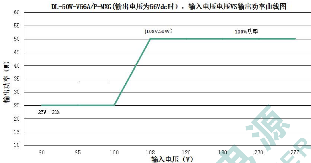
DL-50W-V56A/P-MXG(输出电压为 56Vdc 时, 不同输入电压对应的额定输出电流值和输出功率)
