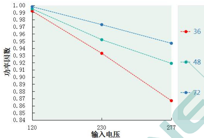
功率因素 VS 输入电压 DL-50W-V72A/P-MXG
