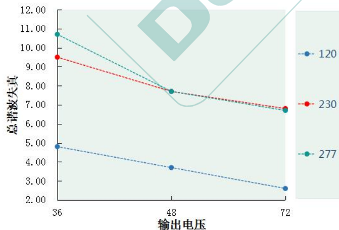
总谐波失真 VS 输出电压 DL-50W-V72A/P-MXG
