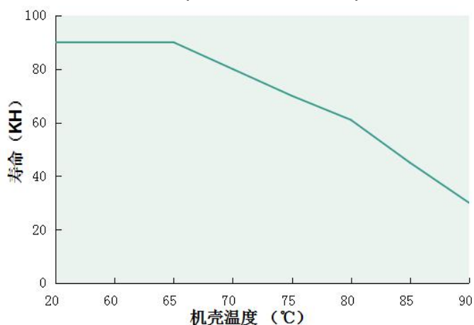
Tc VS 寿命(DL-50W-A/P-MXG)
