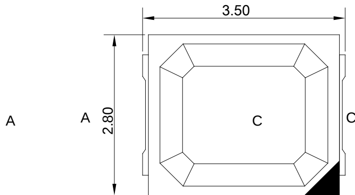
Fig.1-1 Top view 正面视图
