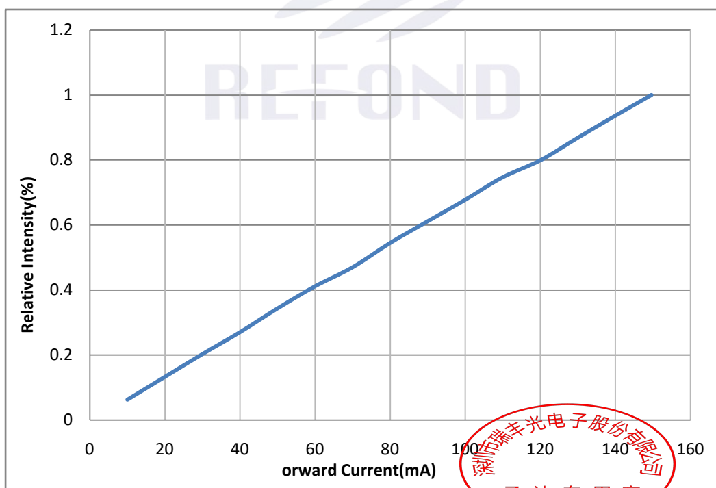
Fig.2- Forward Current Vs. Relative Power 正向电流与相对光功率特性曲线
