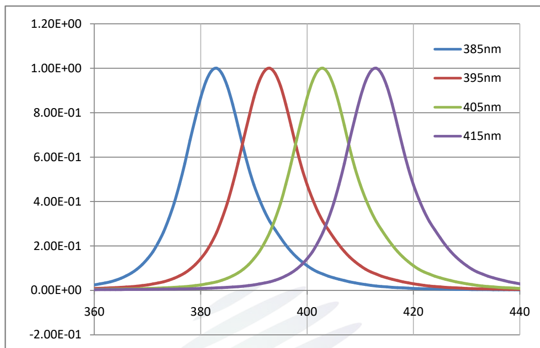
Fig.5-Spectrum Distribution 光谱分布特性曲线
