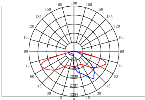
配光曲线
