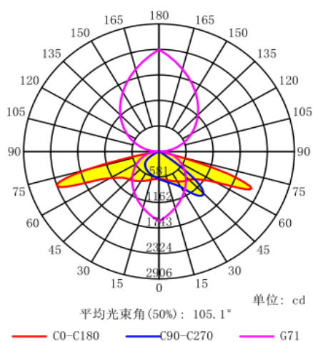
配光曲线
