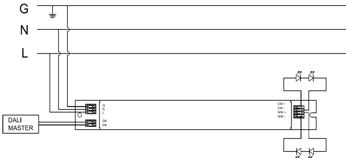
Fig.A:Dali Dimming
