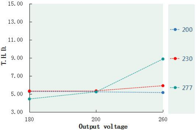
T.H.D. VS Output voltage(DL-240H-PXC)
