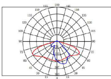
配光曲线
