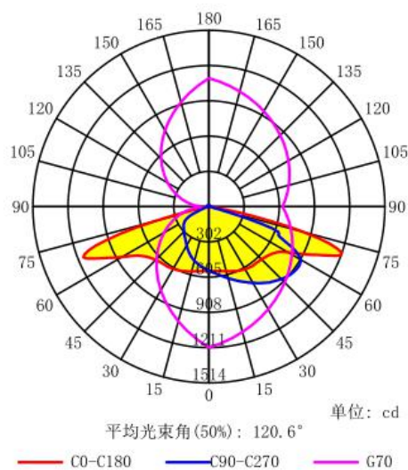
配光曲线
