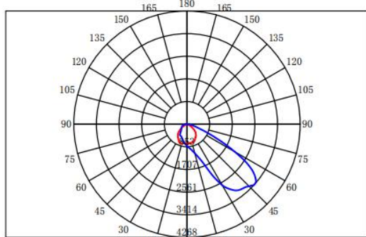
配光曲线
