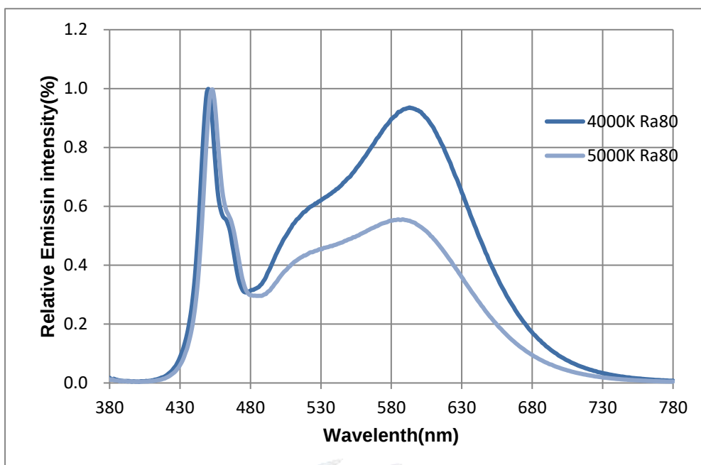
Fig 1-12 Spectrum Distribution 光谱分布特性曲线
