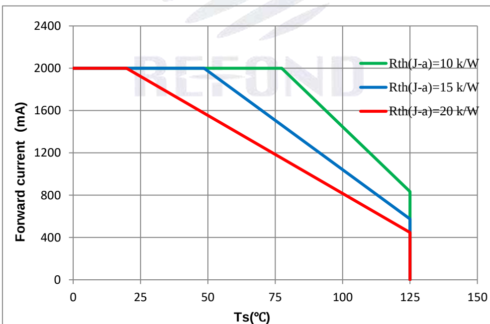
Fig 1-10 Ts Temperature Vs Forward Current 管脚温度与正向电流特性曲线
