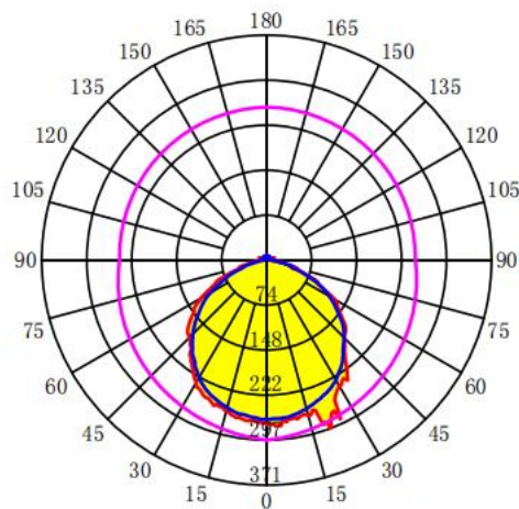
配光曲线
