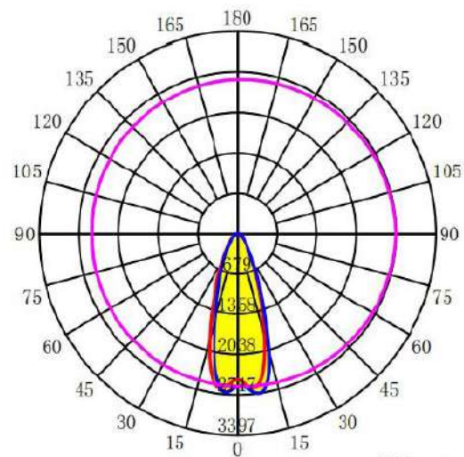
配光曲线
