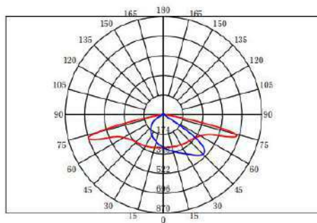
配光曲线
