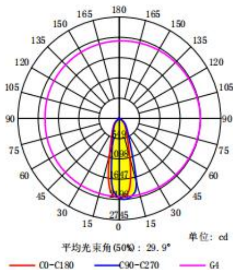
配光曲线
