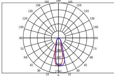
配光曲线
