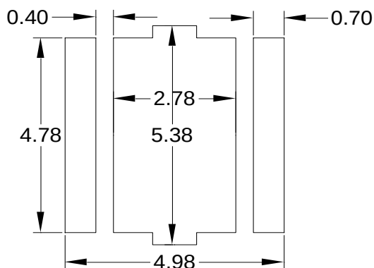
Fig.1-11 Soldering patterns 推荐焊盘 (常规 6V 使用)
