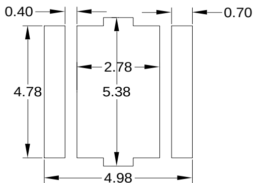
Fig.1-6 Soldering patterns 推荐焊盘 (常规 3V 使用)
