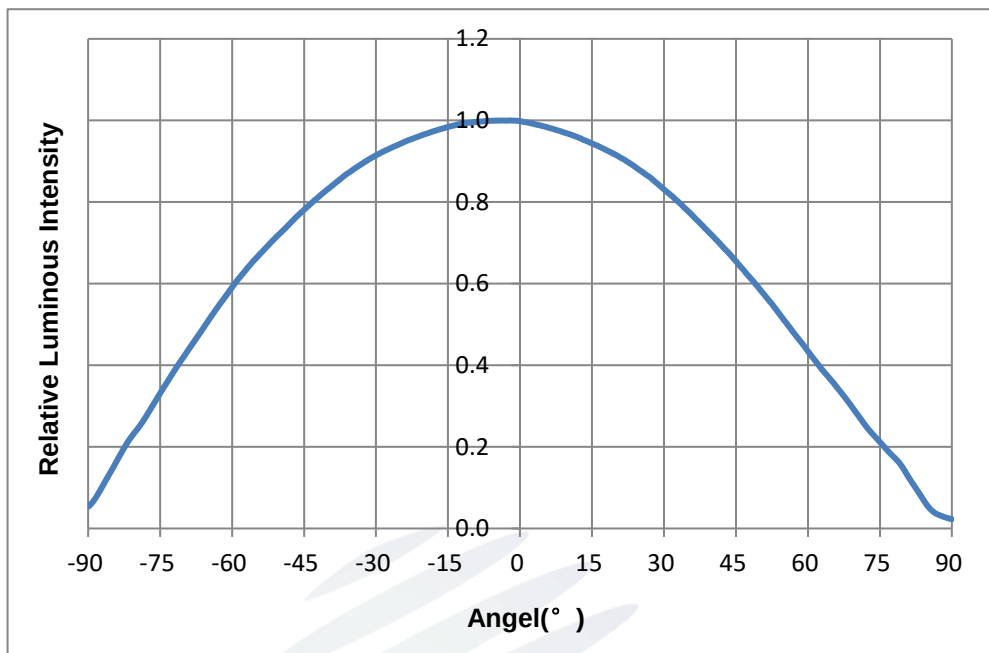
Fig 1-23 Radiation diagram 辐射特性曲线
