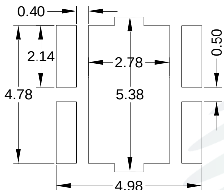
Fig.1-8 Soldering patterns 推荐焊盘 (跳线 6V 使用)
