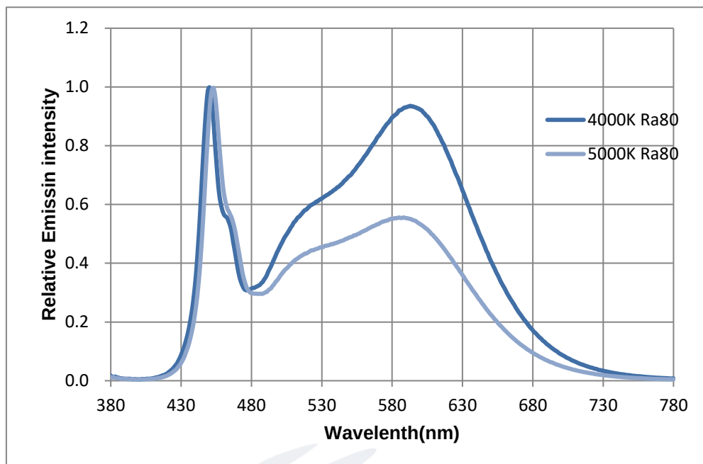
Fig 1-24 Spectrum Distribution 光谱分布特性曲线
