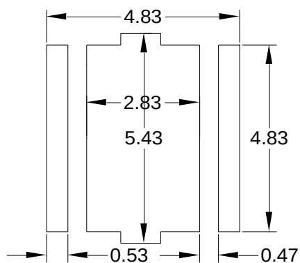
Fig.1-16 Soldering patterns 推荐焊盘 (常规 12V 使用)
