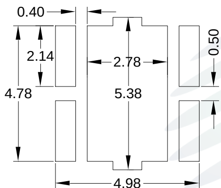
Fig.1-13 Soldering patterns 推荐焊盘 (跳线 12V 使用)
