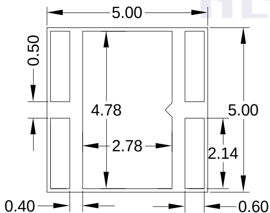
Fig.1-10 Bottom view 背面视图
