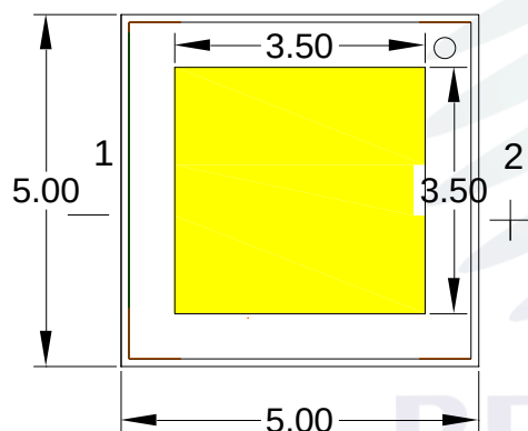
Fig.1-3 Top view 正面视图
