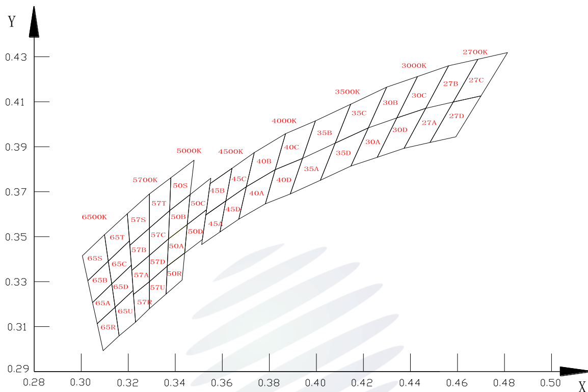
Fig.1-18 Chromaticity Coordinates 色坐标图
