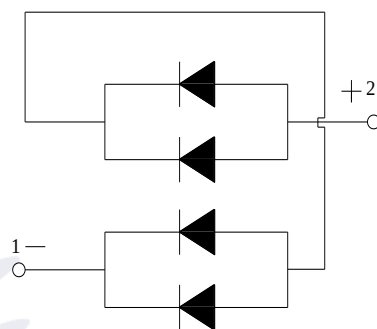
Fig.1-9 Polarity 极性 (跳线 6V 使用)
