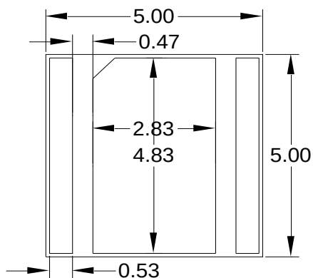
Fig.1-15 Bottom view 背面视图
