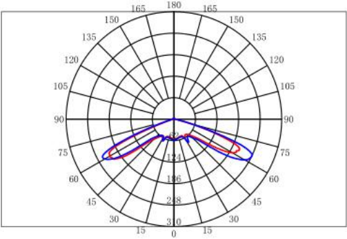
配光曲线
