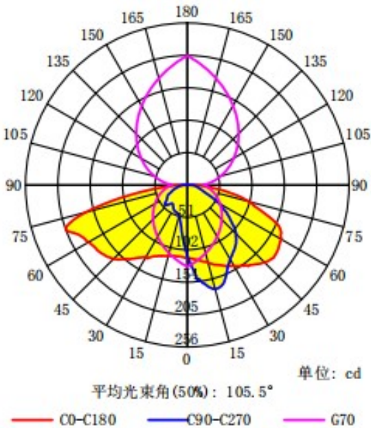
配光曲线
