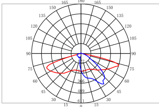
配光曲线
