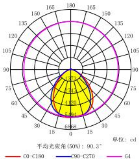
配光曲线
