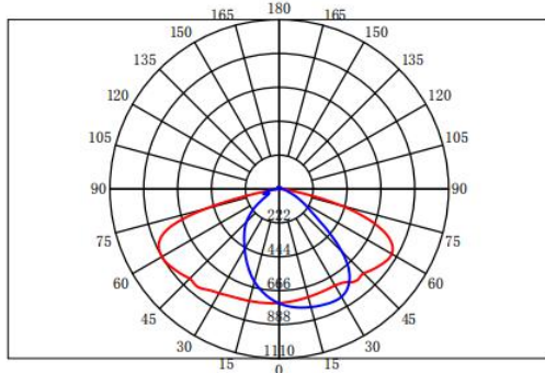
配光曲线
