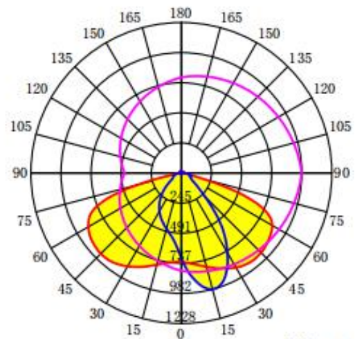
配光曲线
