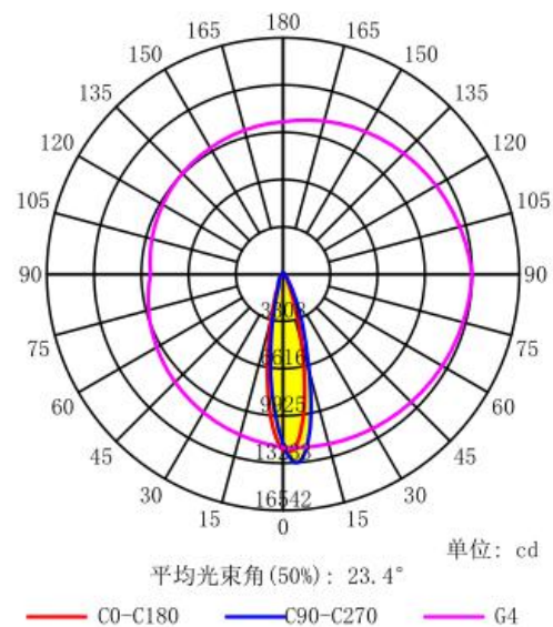
配光曲线
