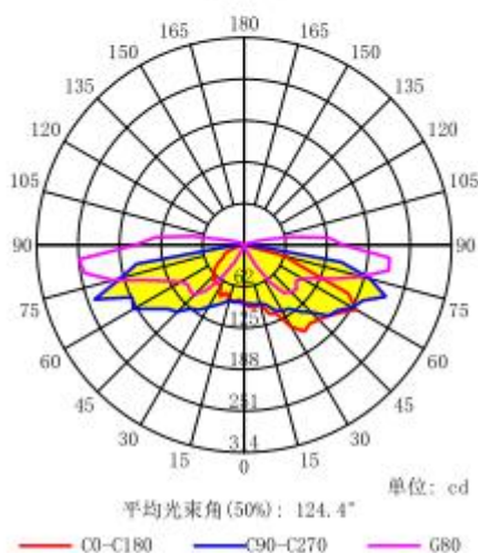
配光曲线
