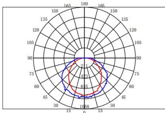
配光曲线
