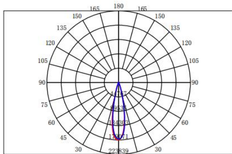
配光曲线
