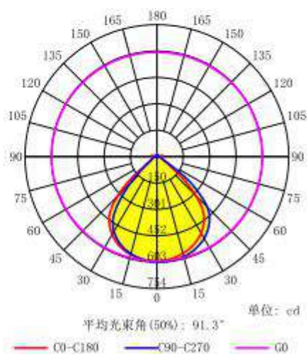
配光曲线
