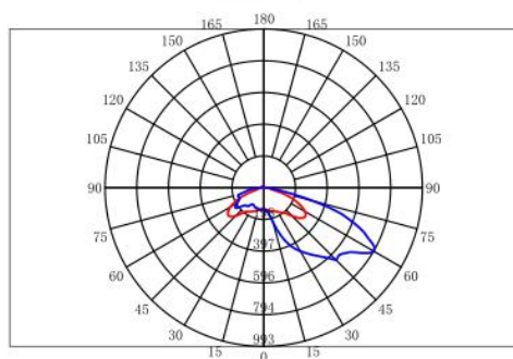
配光曲线
