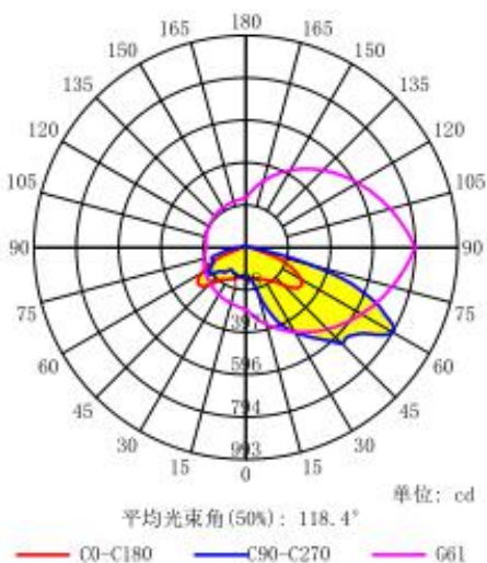
配光曲线
