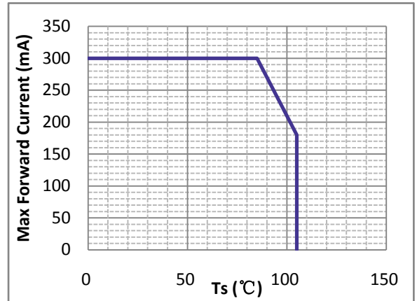
Max. forward current vs. T_s temperature 最大电流与 T_s 特性曲线 ( T_j \leq 125^\circ\text{C} )
